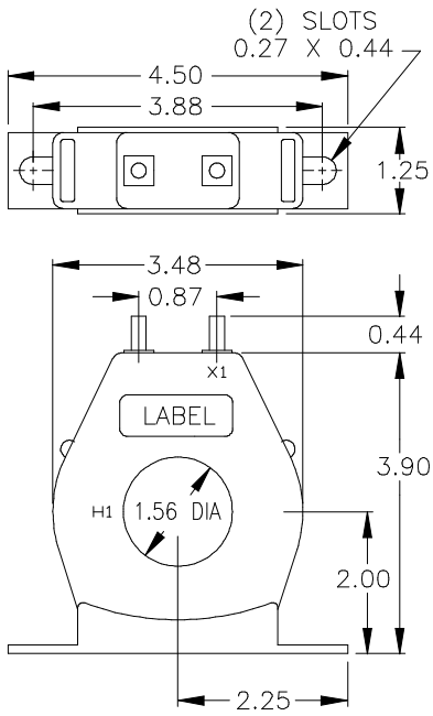
Model 5RBT
